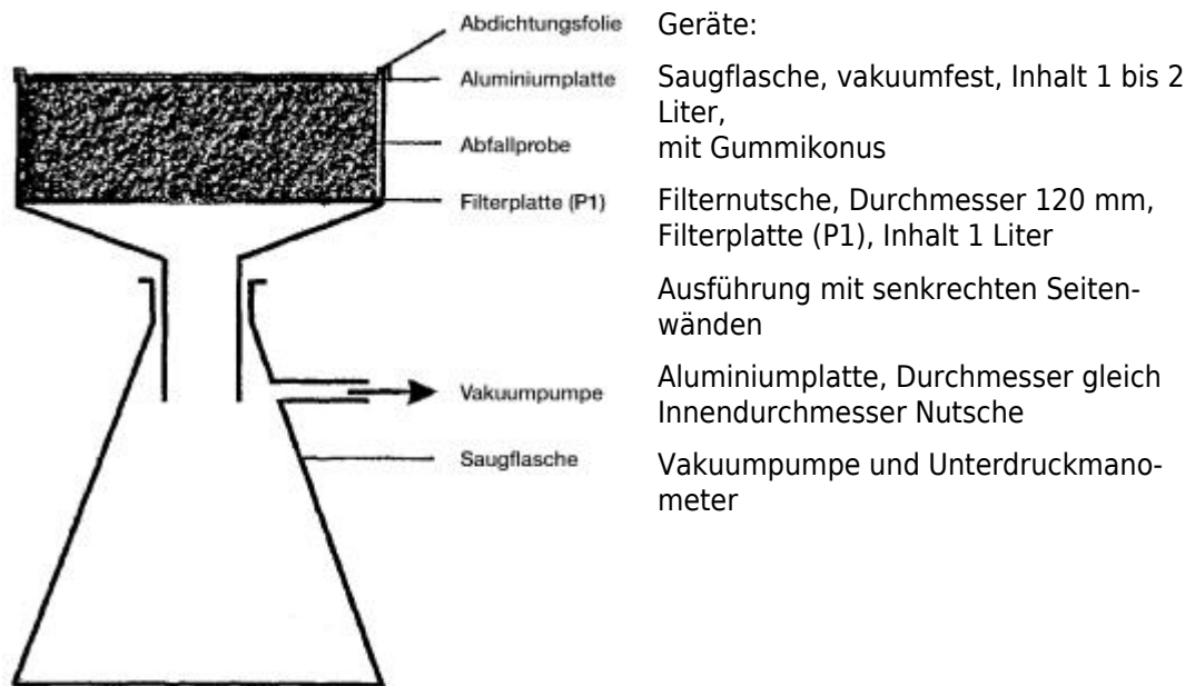
Bild 1: Apparatur zur Einstellung des Wassergehaltes
